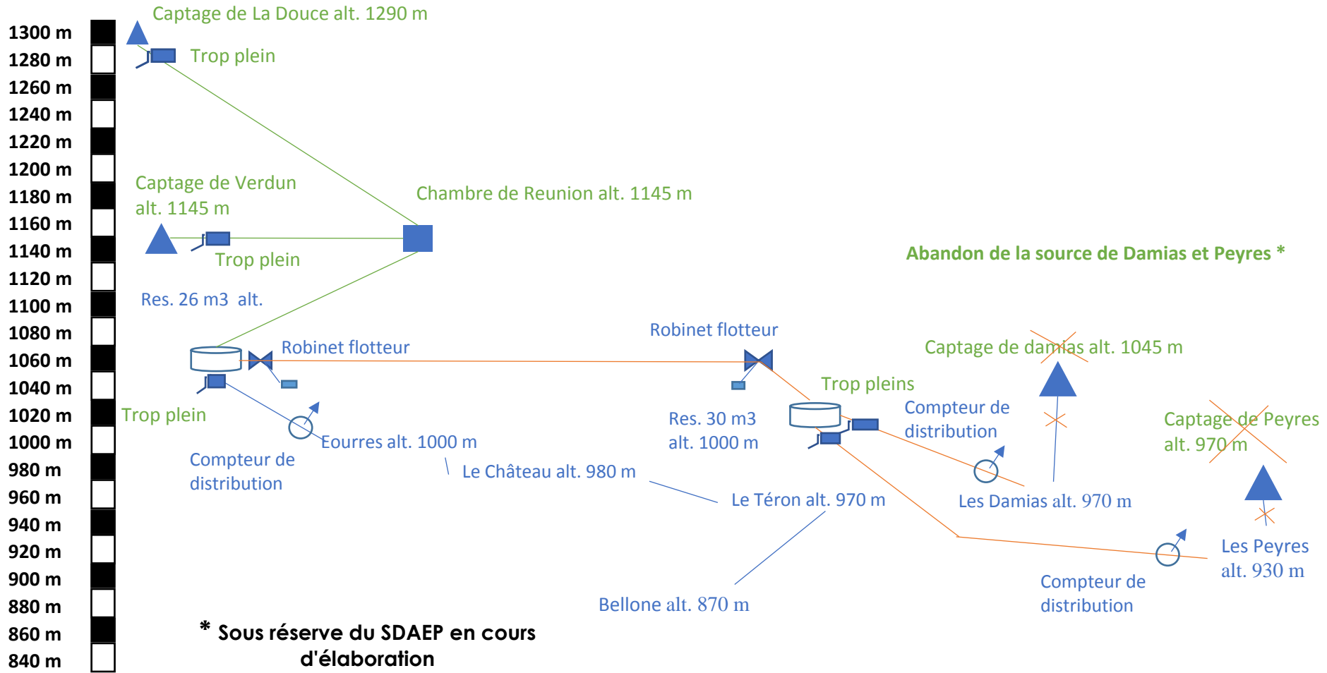
Planche graphique n°4 BIS : Synoptique du réseau futur *
